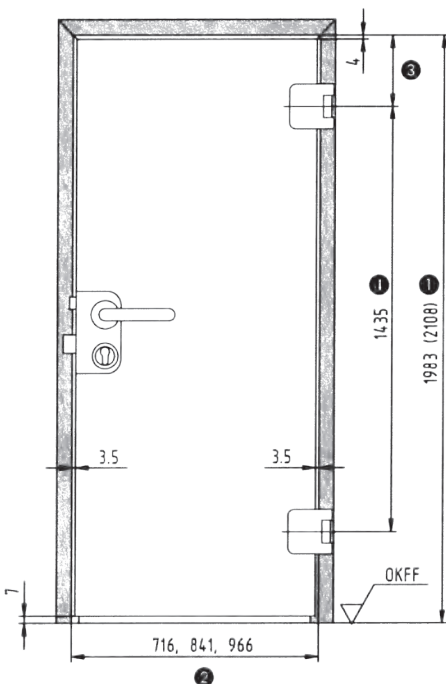
Standard-Glastürblatt mit Zarge
